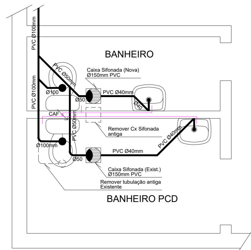
BANHEIROS PLANTA BAIXA Escala 1:25
